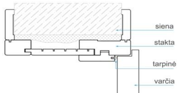
Reguliuojamos staktos matmenys (mm):
